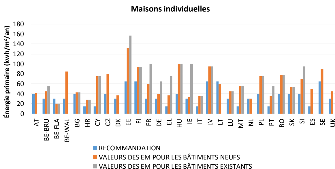
Graphique 4: Comparaison indicative des définitions des bâtiments dont la consommation d'énergie est quasi nulle avec les critères de référence recommandés par la Commission, pour les maisons individuelles
