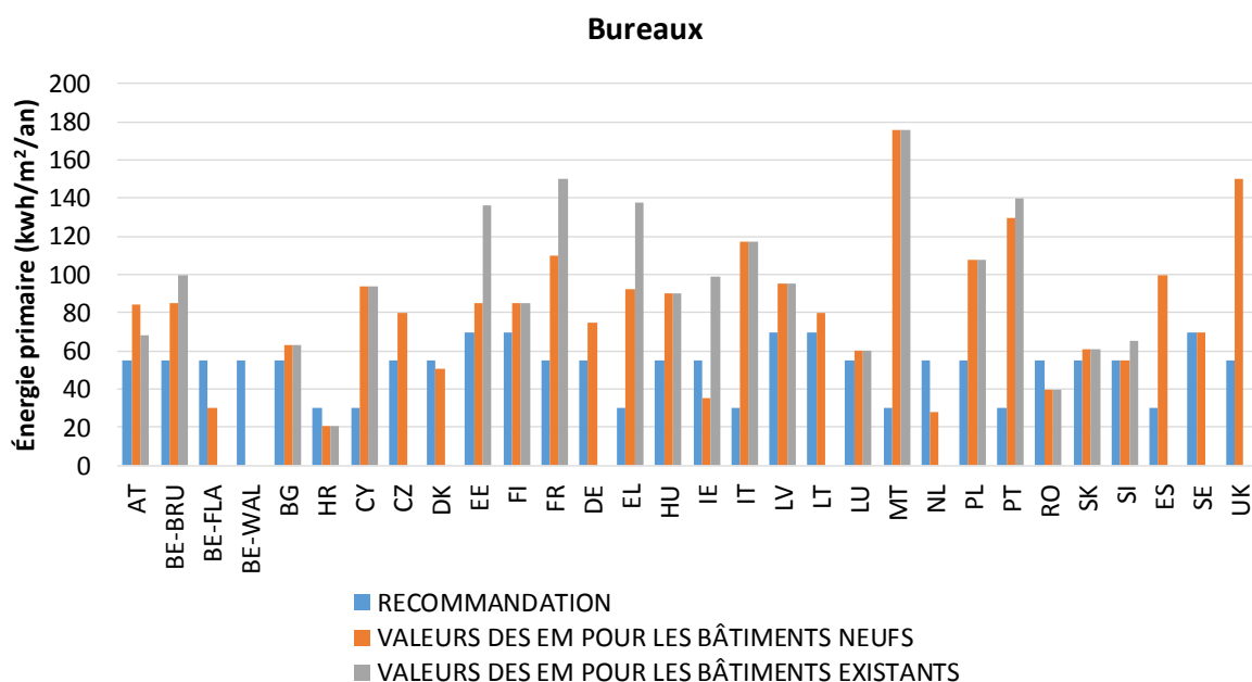
Graphique 5: Comparaison indicative des définitions des bâtiments dont la consommation d'énergie est quasi nulle avec les critères de référence recommandés par la Commission, pour les bureaux
